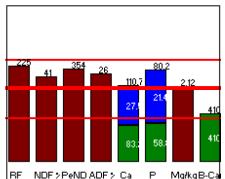
Struktur / Mineralstoffe
